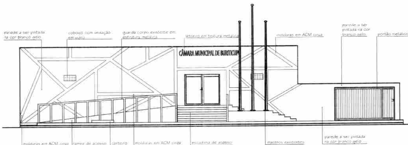
FACHADA esc. 1:100
